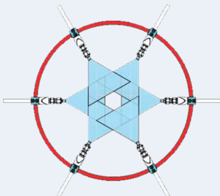
Anel de pulverização de 6 bicos para tubos de 5 a 8 OD
