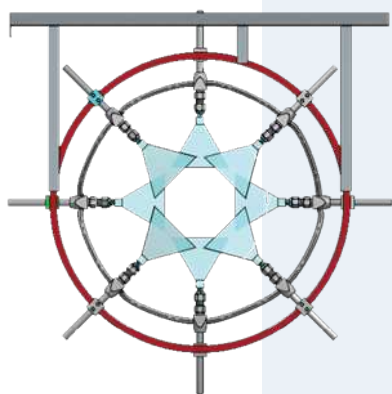
Anel de pulverização de 8 bicos para tubos de 9 a 12 OD
